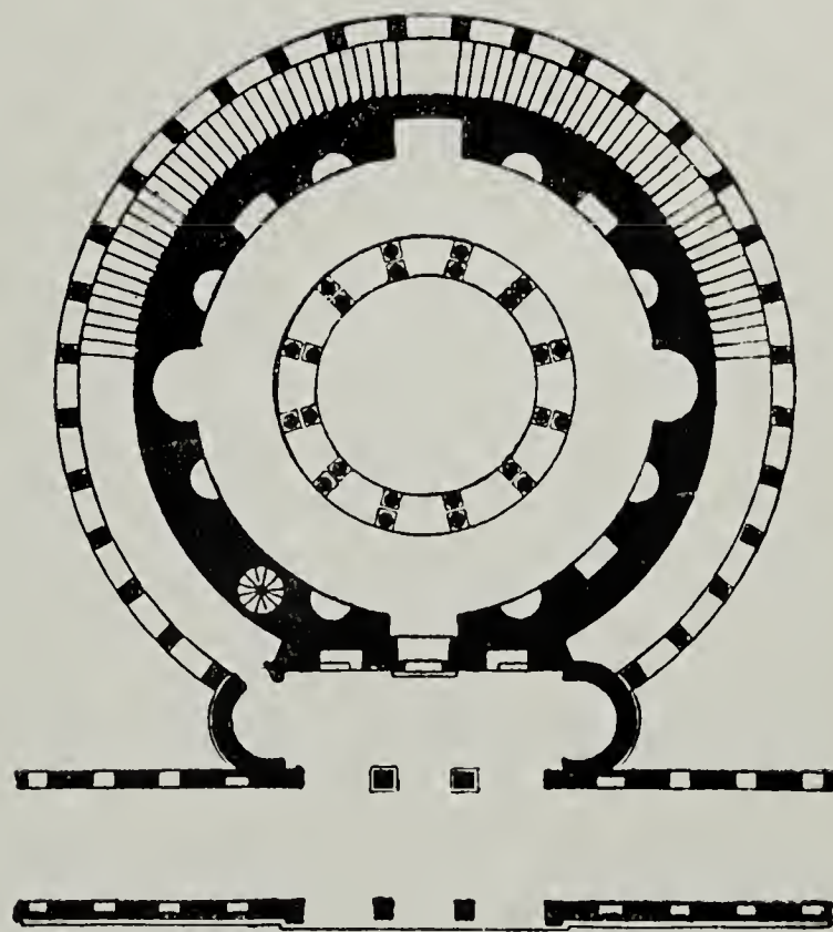
Figura 44 —Planta del mausoleo de Constanza (Iglesia de Santa Constanza) en Roma.
